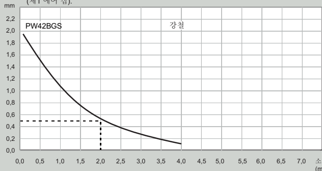
▲ 센서와 첫 번째 판재 사이의 최대 에어 갭 (제1 에어 갭).
