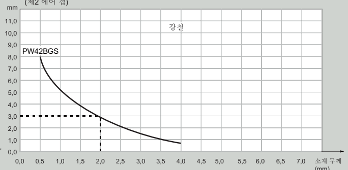
▲ 첫 번째 판재와 두 번째 판재 사이의 최대 에어 갭 (제2 에어 갭).
